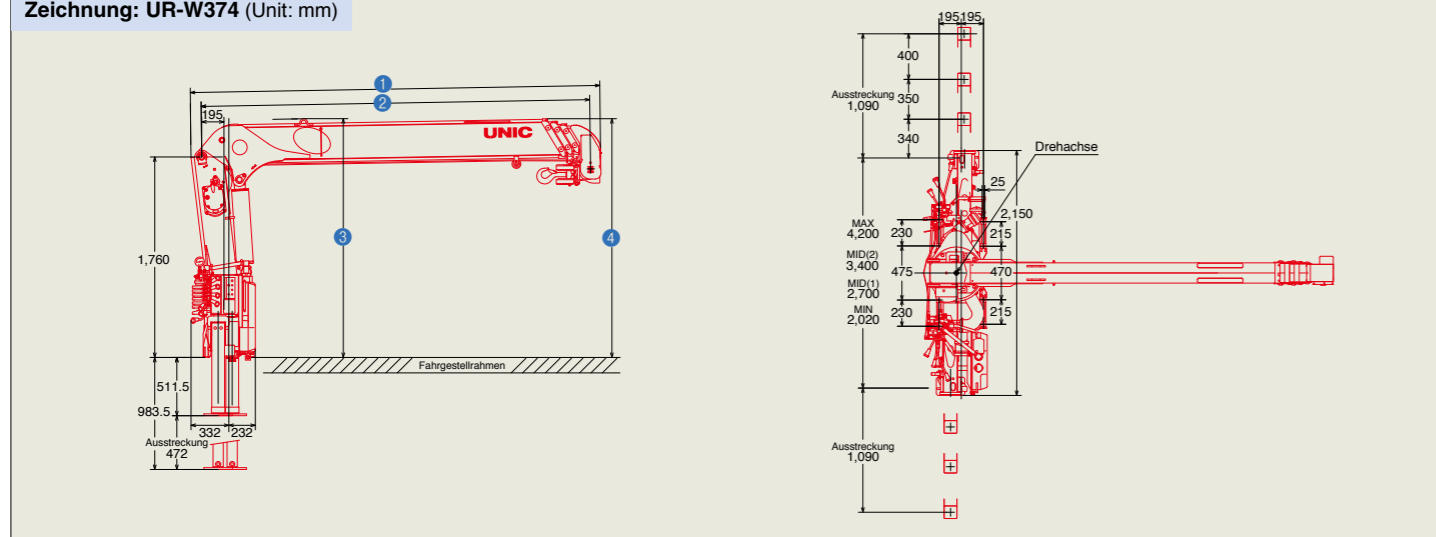
Zeichnung: UR-W374 (Unit: mm)
